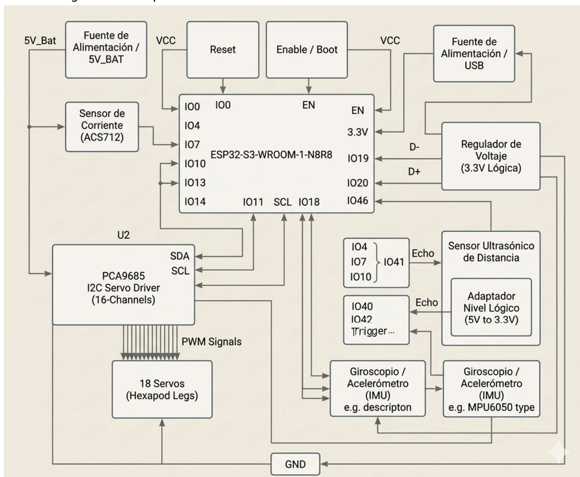
Diagrama de bloques del sistema
